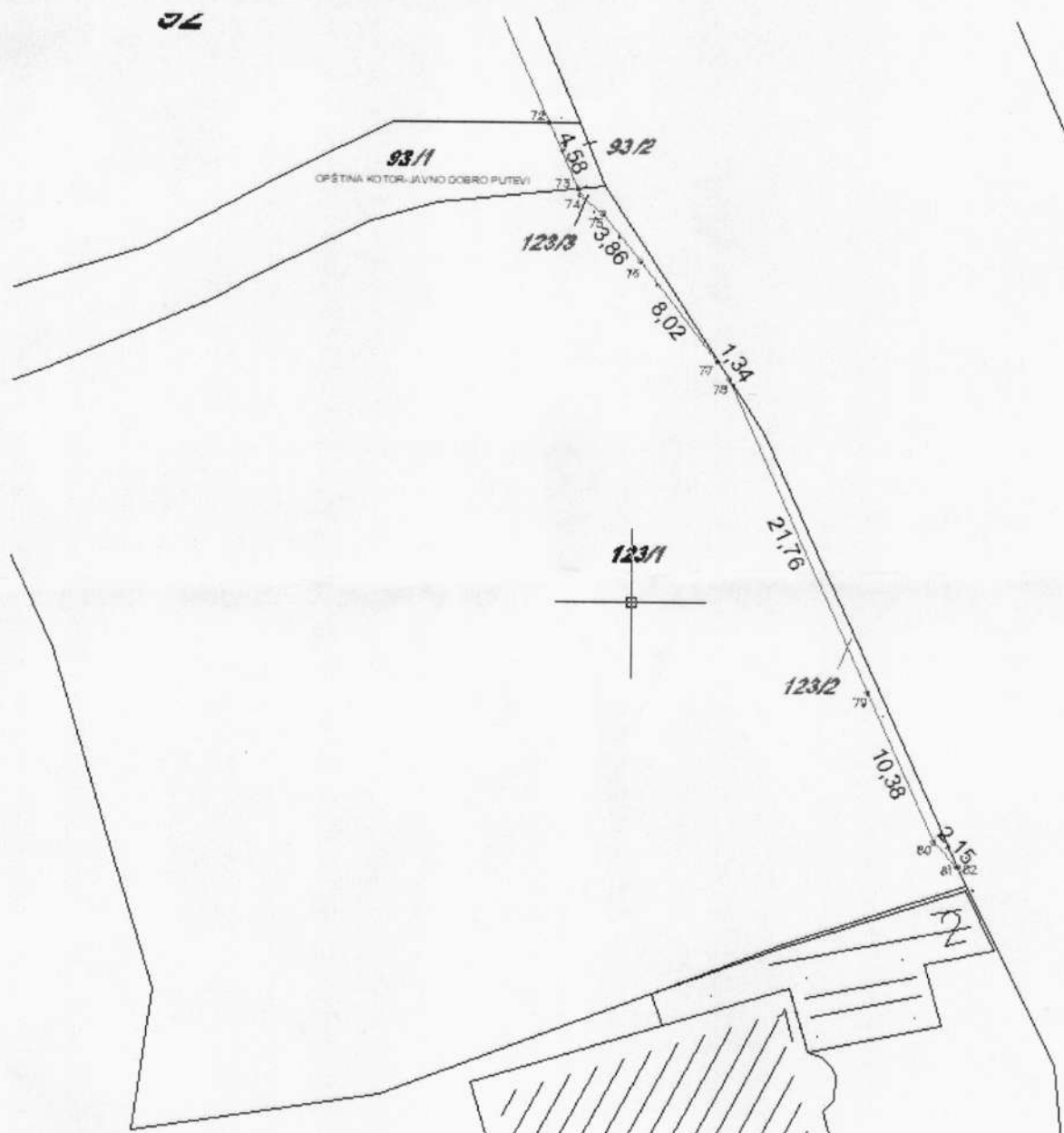
Skica katastarske parcele 123 KO Kubasi
